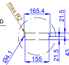
Dettaglio D Scala 1:7
